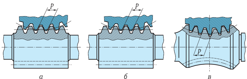
2.5-Сурет. (а) архимедті, (б) эвольвентті және (в) глободті бұрамдықты бар бұрамдықты берілістердің сызбалары:
