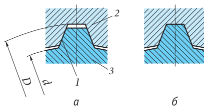
1.12-Сурет. (а) білік дөңестерінің бүйір қырлары бойынша орталыққа келтіре отырып эвольвентті ойма кілтекті жалғаужәне (б) оның сыртқы диаметрі бойынша жалғау: 1 — эвольвент; 2 — күпшек; 3 — білік; d , D — біліктің ішкі және сыртқы диаметрлері
