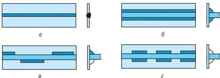
1.32-Сурет. Ұзындығына қарай дәнекерлеп жапсарлай отырып жалғаудың жіктелуі:
